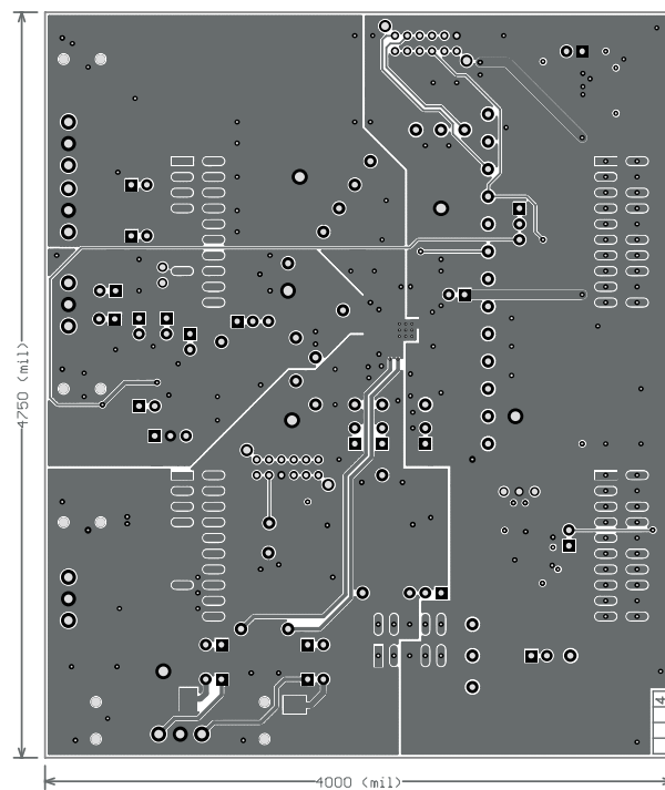
Figure C-4. Bottom Layer
